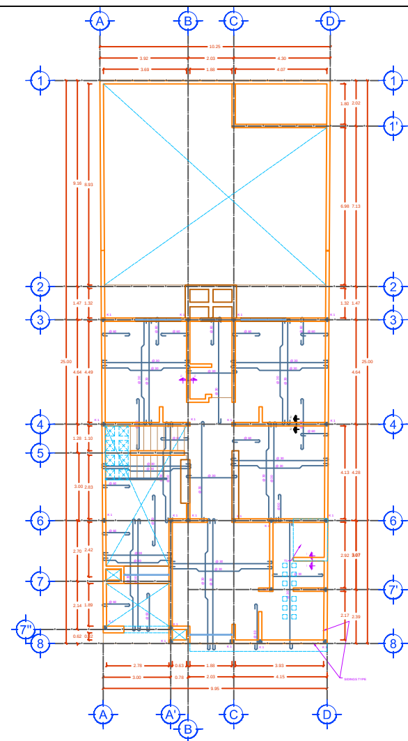
STRUCTURAL PLAN SCALE: 1:100
