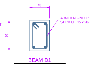
BEAM D1
